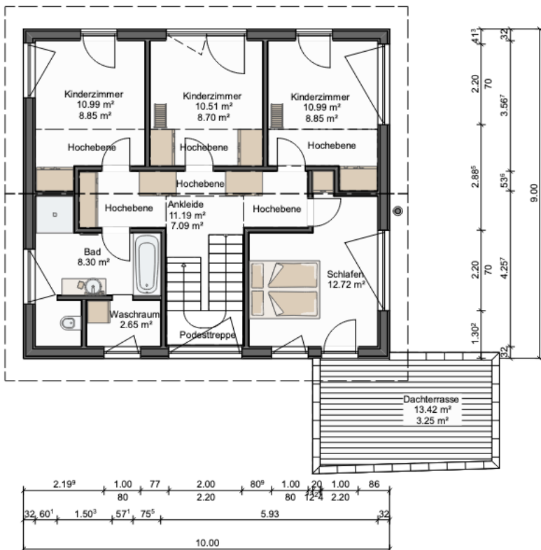
Dachgeschoss M 1: 100
